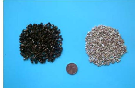
Abbildung 1: menex ® ™ -POMS vor (links) und nach (rechts) Durchströmung von.
